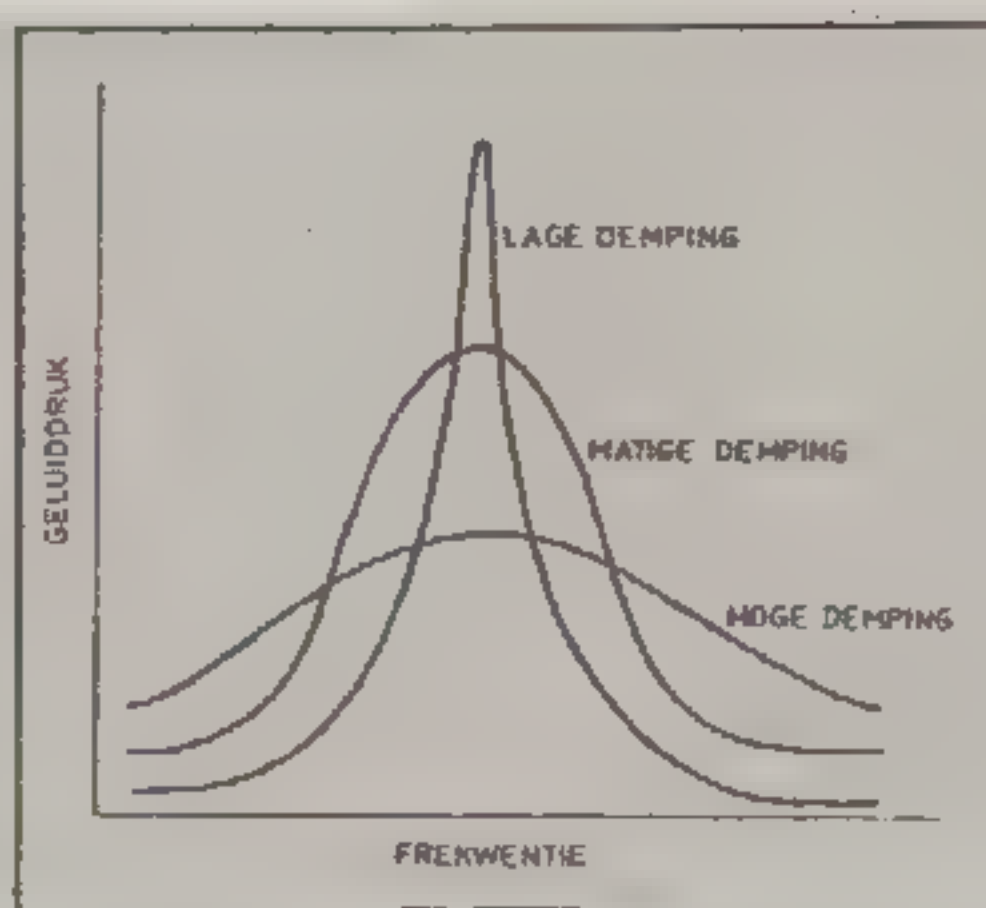
fig. 10 Invloed van demping op een resonantie
